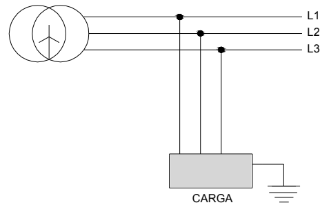
Figura 5 - Esquema IT
